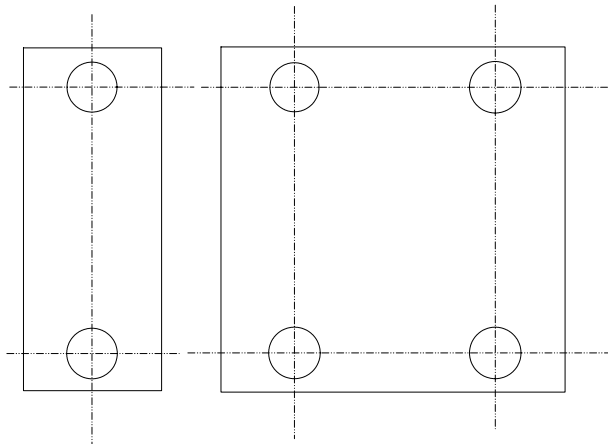
Ankerplatte, verschiedene Maße und Ausführungen möglich Abhängig von Belastung und Wandbeschaffenheit
