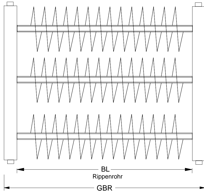
Rippenrohrregister 3-lagig mit Sammler
